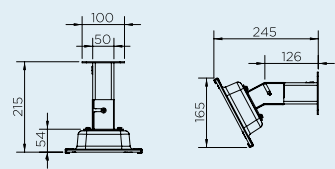
MEDIDAS DEL SOPORTE
