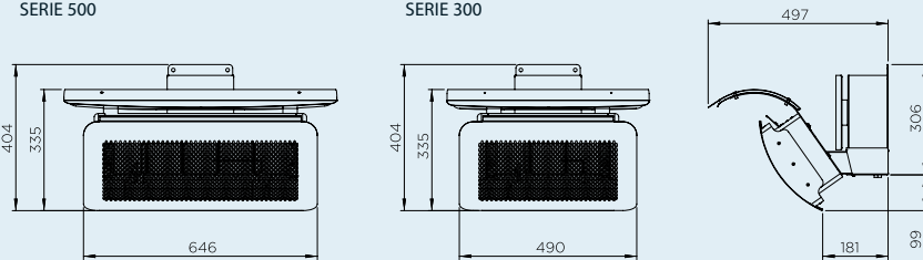
MEDIDAS DEL PRODUCTO CON DEFLECTOR DE CALOR SERIE 500
