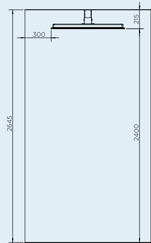
SEPARACIÓN DE MONTAJE DE TECHO
