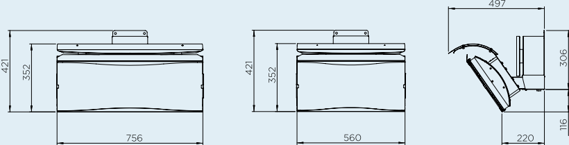
MEDIDAS DEL PRODUCTO CON DEFLECTOR DE CALOR SERIE 500
