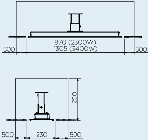
CAVIDAD MÍNIMA OPCIÓN 1
