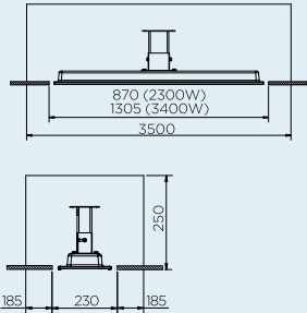
CAVIDAD MÍNIMA OPCIÓN 2
