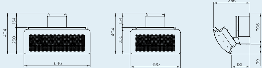
MEDIDAS DEL PRODUCTO SERIE 500
