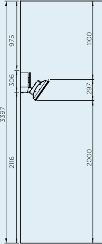
SEPARACIÓN DE MONTAJE EN PARED
