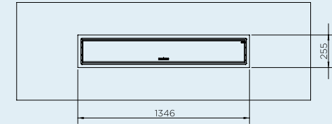
MARCO DE MONTAJE EMPOTRADO EN EL TECHO 3400 W
