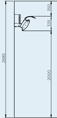
SEPARACIÓN DE MONTAJE EN PARED CON DEFLECTOR DE CALOR
