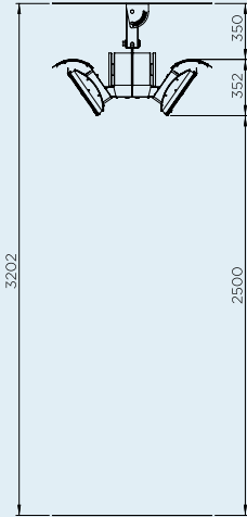
SEPARACIÓN DE POSTE DE TECHO CON DEFLECTOR DE CALOR
