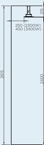
MONTAJE EN PARALELO AL SUELO
