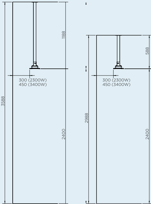
SEPARACIÓN DE POSTE DE TECHO
