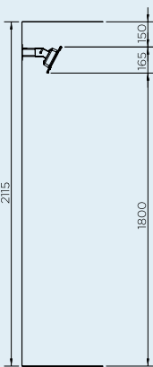
SEPARACIÓN DE MONTAJE EN PARED
