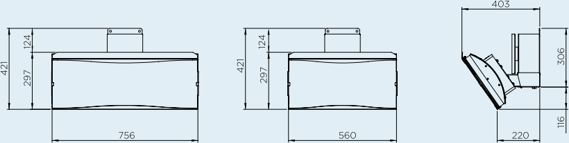
MEDIDAS DEL PRODUCTO SERIE 500
