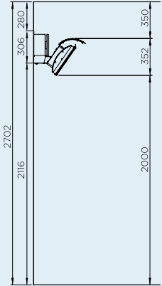
SEPARACIÓN DE MONTAJE EN PARED CON DEFLECTOR DE CALOR
